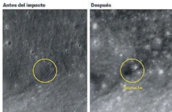
Imagen tomada por Danuri de la Luna antes y después del impacto.
